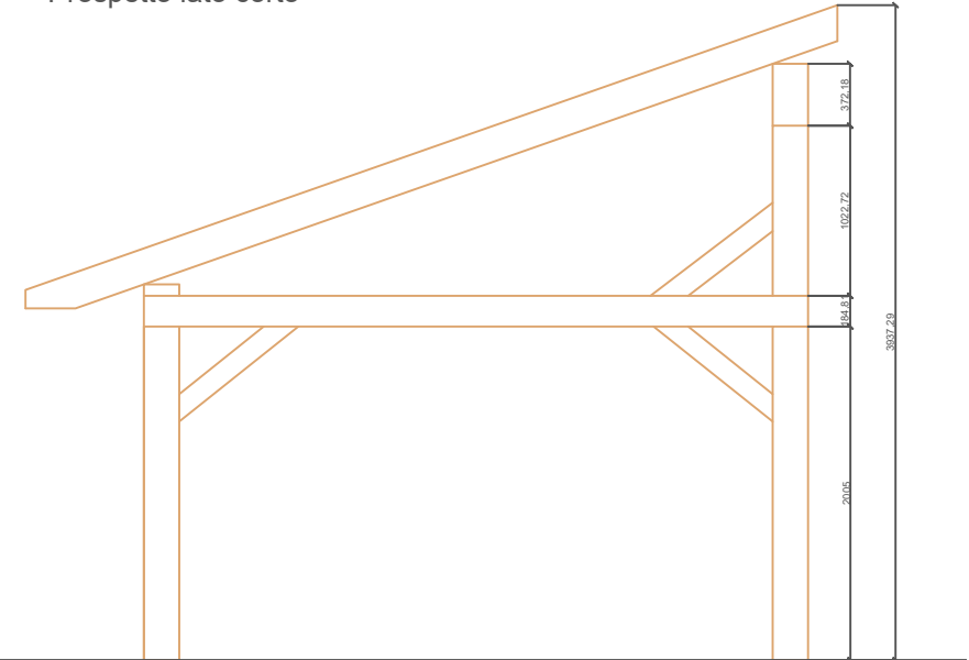
Prospetto lato corto
